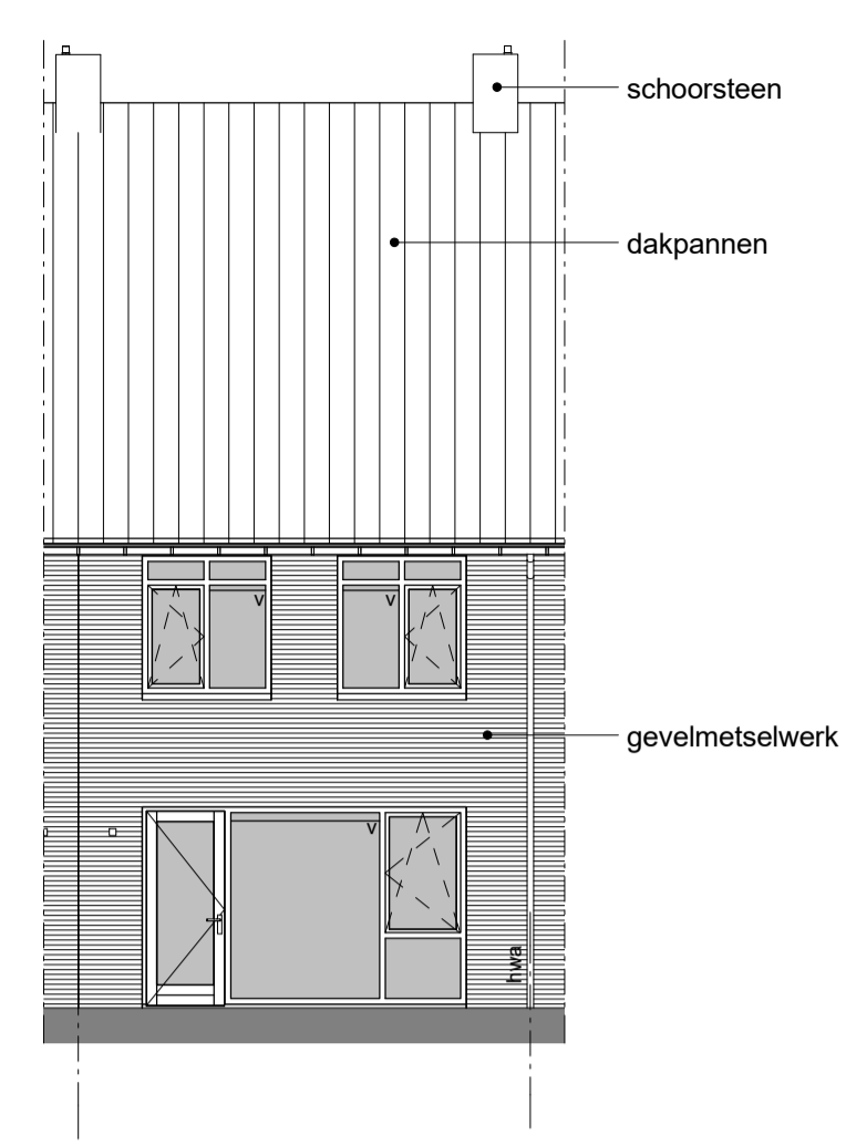
ACHTERGEVEL - 1:100
