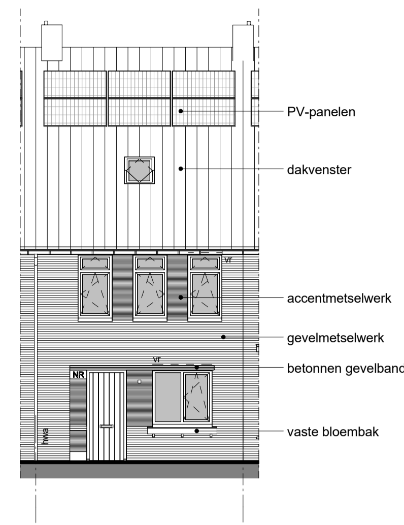
VOORGEVEL - 1:100
