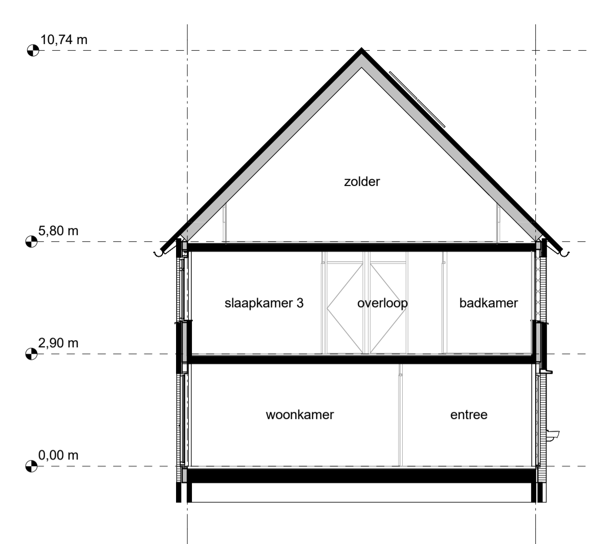
DWARSDOORNSEDE - 1:100
